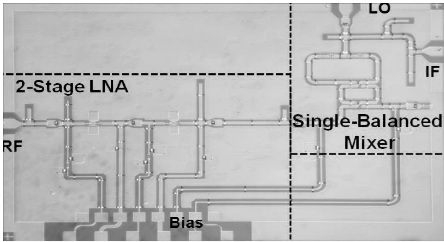
▲ 위의 칩은 레이더의 부품인 소음 감속 LNA와 Mixer를 합친 것이다.
