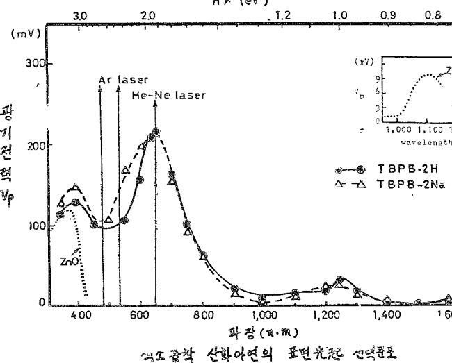
가시광 및 근적외광의 화상 기록 특성에 대한 그래프
